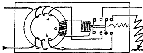
Bild 2b: Gegenwart eines Isolationsfehlers in der Isolation (zwischen einem Leiter und der Erde)
