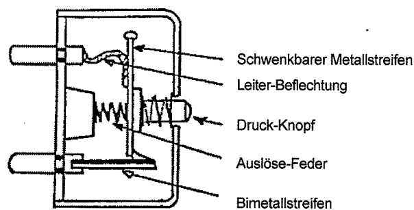
Bild 1: Thermischer Schutzschalter
