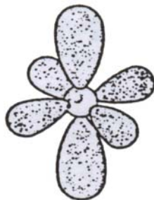
sp^3 -Hybridorbital
