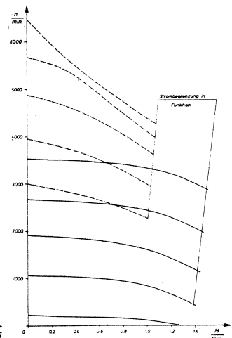
Drehzahl-Drehmoment-Kennlinie MEL 4 000
