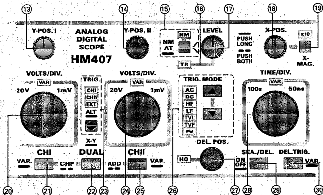
(26) TRIG. MODE - Drucktasten mit LED's.
