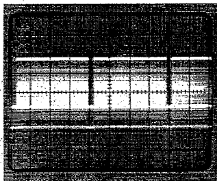
Bild 3 MODE: DEL (DELAY = verzögern) TIME / DIV. : 5ms/cm Triggerkopplung: TV-F Triggerflanke: fallend (-) Verzögerungszeit: 4cm x 5ms = 20ms
