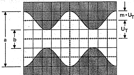
Figur 2 Amplitudenmodulierte Schwingung:
