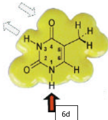
Figur 6. Darstellungen des Thymin.
