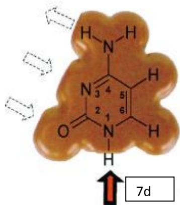
Figur 7. Darstellungen des Cytosin.
