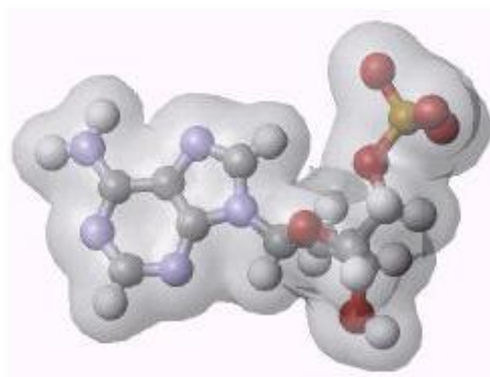
Figur. 12 Darstellungen der Desoxyadenosin 5'Phosphat.
