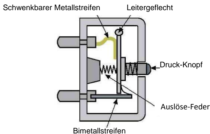
Bild 1: Thermischer Schutzschalter
