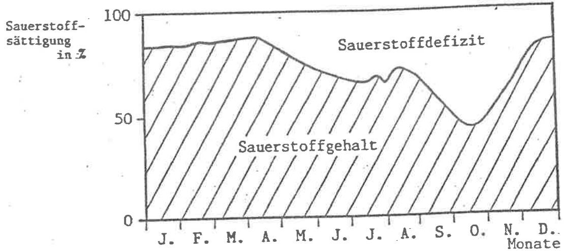
Abb.20: Jahresverlauf (Mittelwert der Jahre 1975-79) der Sauerstoffsättigung eines Flusses (Fulda im Schlitzerland) (nach Brehm 1982)
